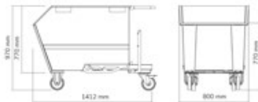
Cuchara portarresiduos basculante capacidad 500 l con ruedas preparada para rejilla y grifo
