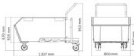
Cuchara portarresiduos basculante capacidad 300 l con ruedas preparada para rejilla y grifo
