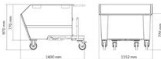
Cuchara portarresiduos basculante capacidad 750 l con ruedas preparada para rejilla y grifo
